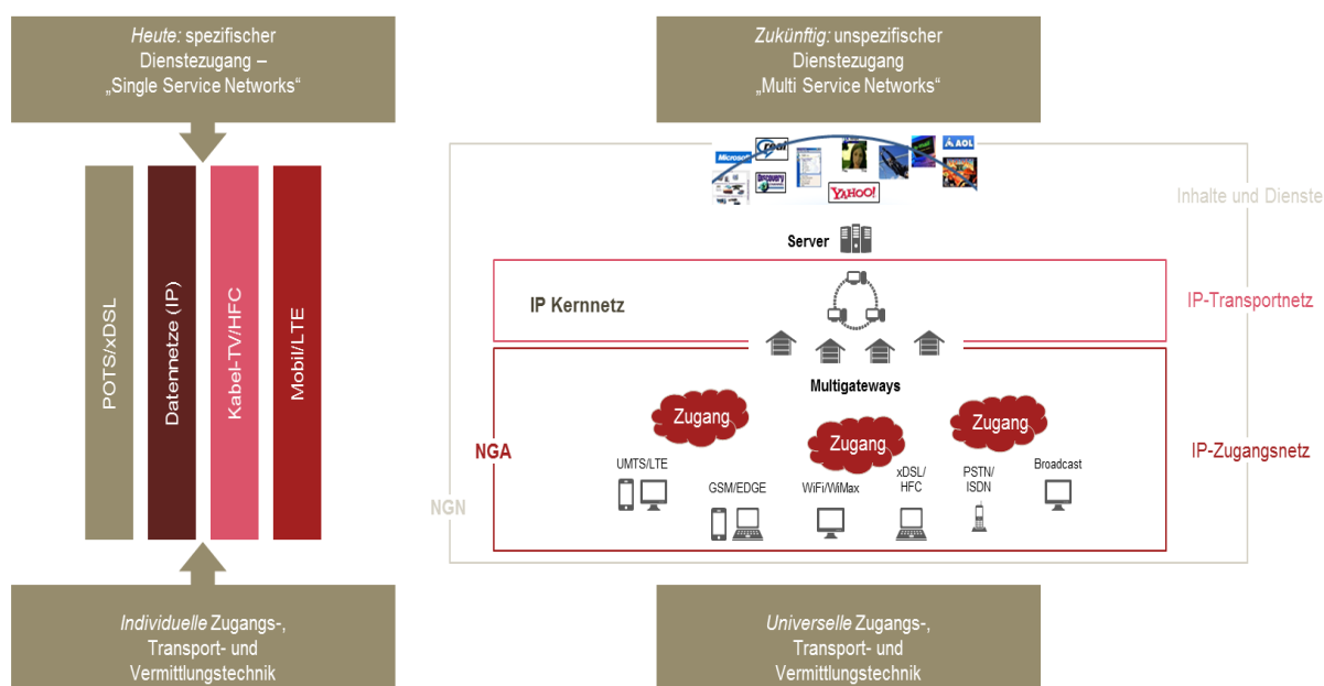
Abbildung 6: Schematische Darstellung heutiger Access-Netze und zukünftiger NGA-Netze in einem vollständigen Next Generation Network.
