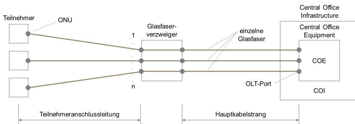
Abbildung 24: Netzstruktur eines optischen Punkt-zu-Punkt-Netzes, [20].
