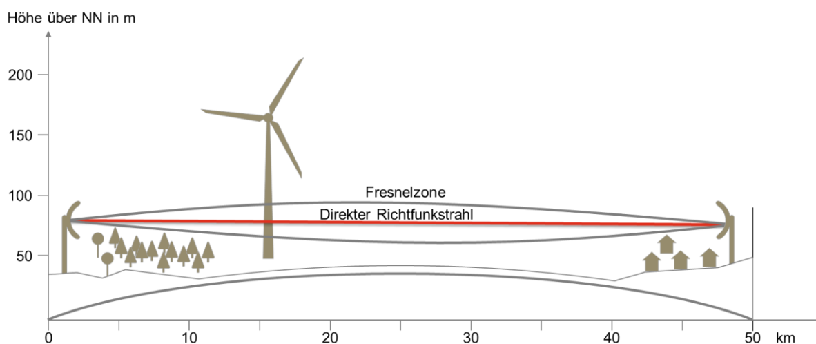
Abbildung 37: Darstellung einer Richtfunkverbindung, [31].
