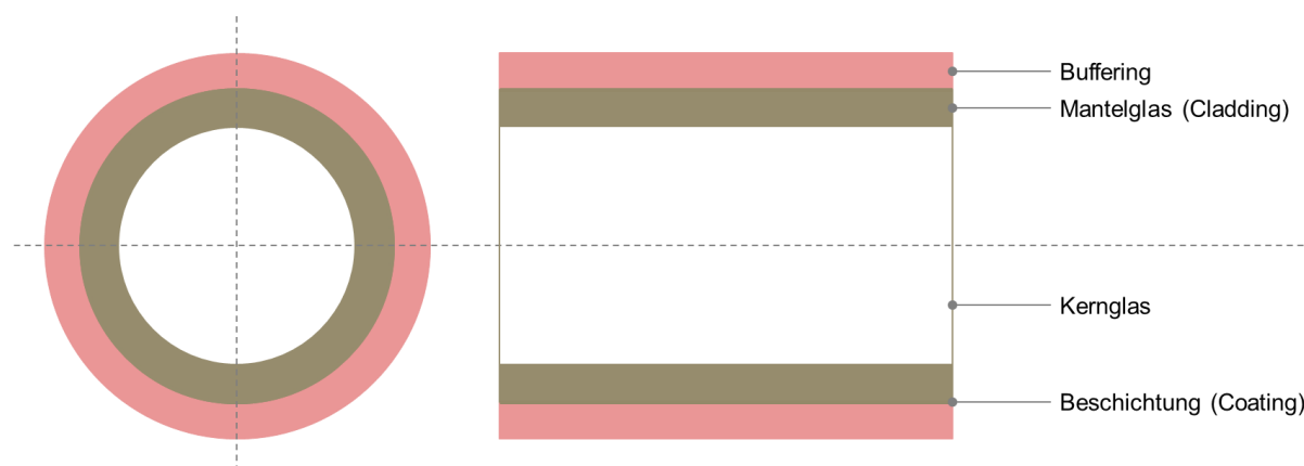
Abbildung 18: Aufbau eines Lichtwellenleiters, [16].
