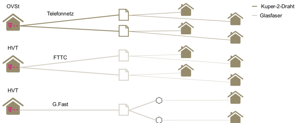
Abbildung 7: Struktur des Kupfer-2-Draht-Netzes mit xDSL-Erweiterungen [2].
