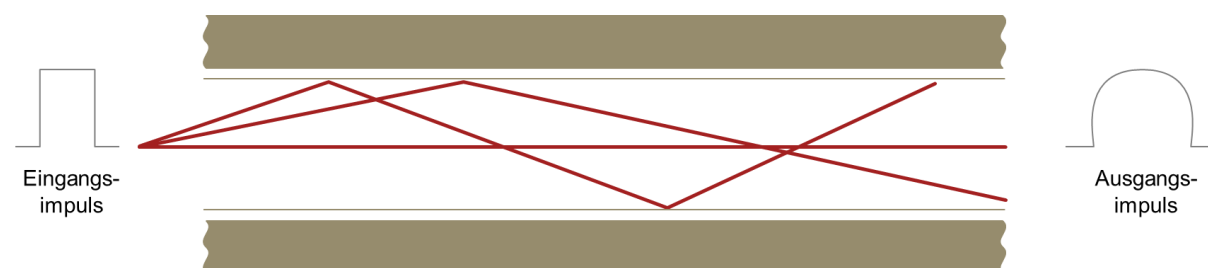
Abbildung 19: Multimodefaser mit Stufenindex-Profil, [16].
