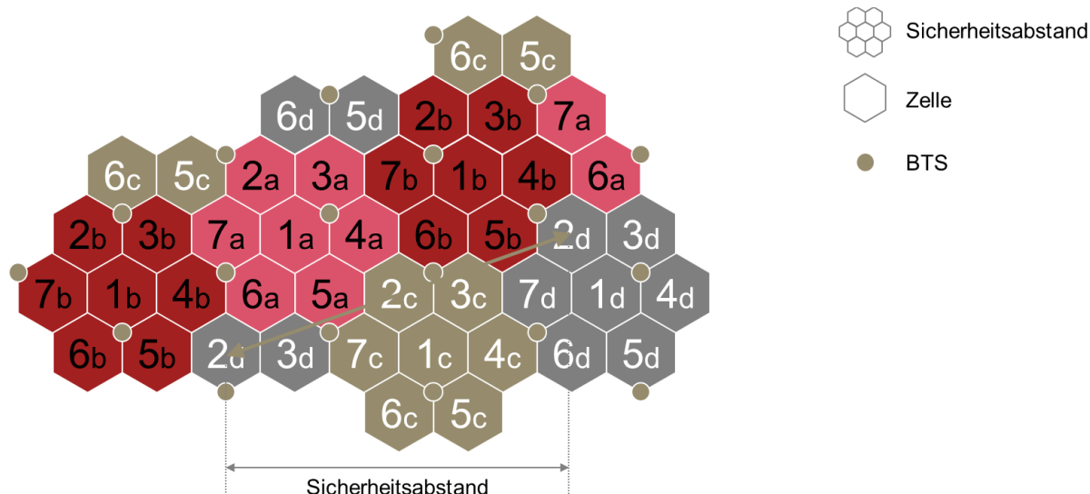
Abbildung 32: Die Abbildung zeigt die grundsätzliche Zellstruktur aktueller Mobilfunknetze am Beispiel von GSM, [24], [25].
