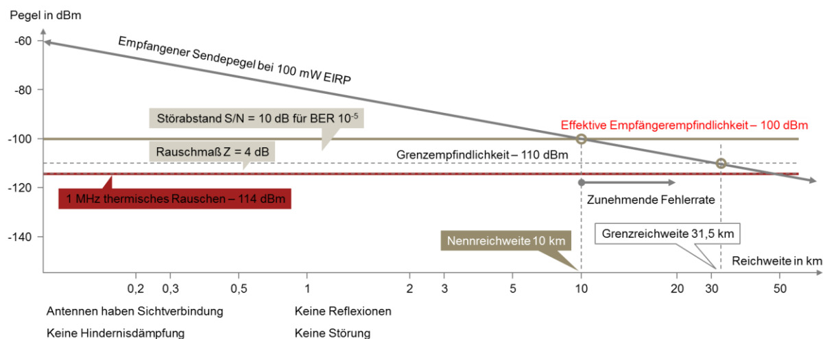
Abbildung 31: Graphische Ermittlung der maximalen Reichweite eines Funksystems [23].
