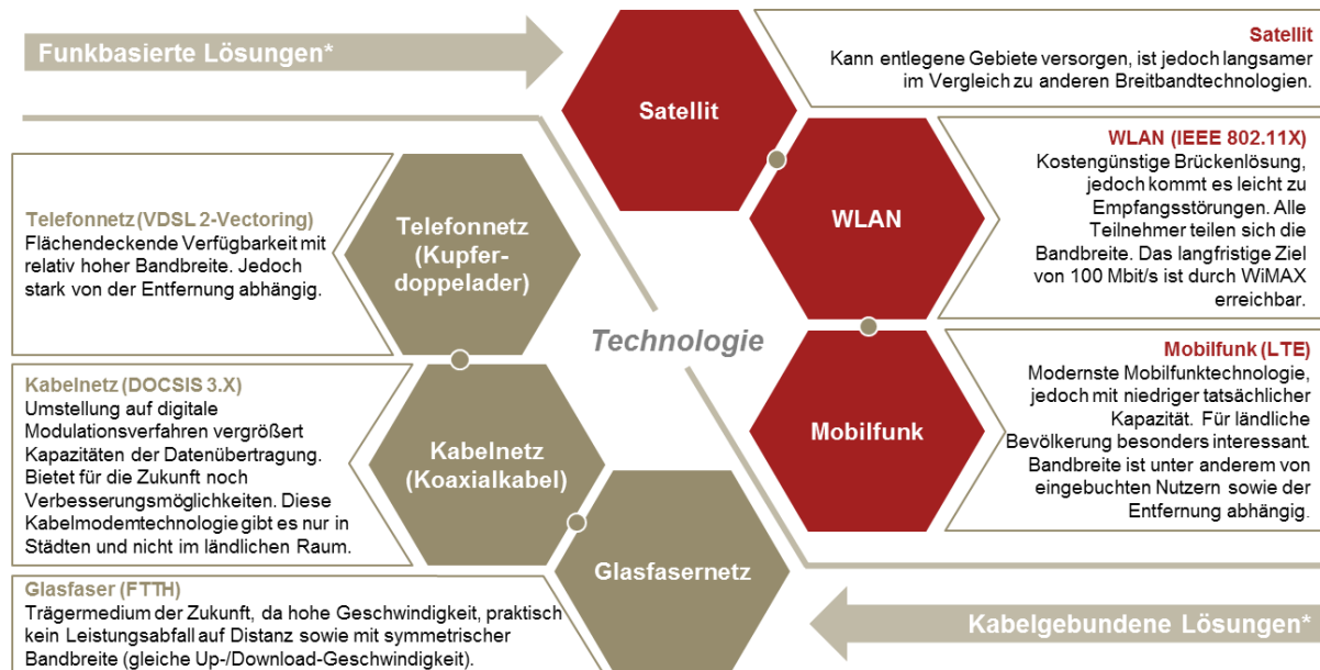
Abbildung 3: Übersicht über kabelgebundene und funkbasierte Übertragungstechnologien.
