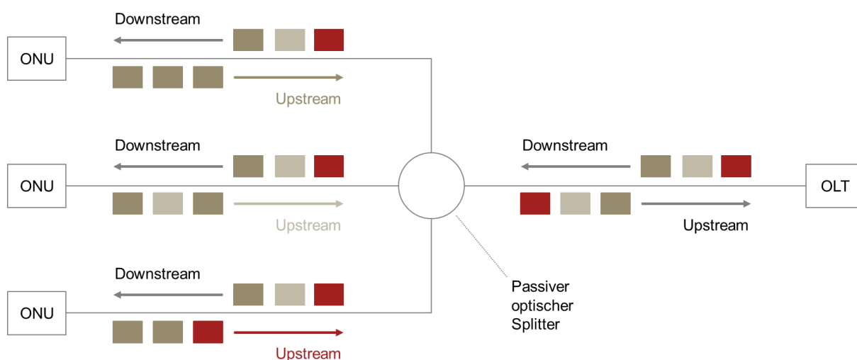
Abbildung 23: Übertragung von Informationen über GPON, [16], [19].
