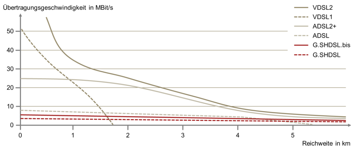
Abbildung 10: Reichweitenabhängigkeit der maximalen Datenrate der unterschiedlichen DSL-Varianten, [4], [5].
