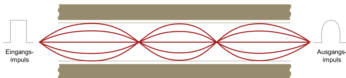
Abbildung 20: Multimodefaser mit Gradientenindex-Profil, [16].
