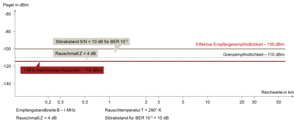
Abbildung 30: Darstellung des thermischen Rauschens und des Empfängerrauschens sowie des Störabstandes [23].
