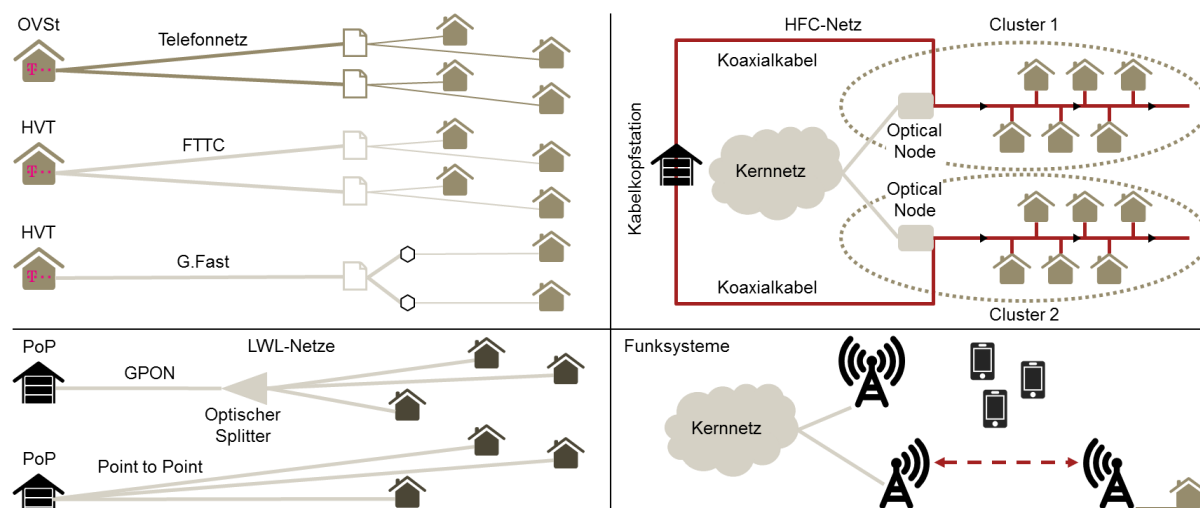
Abbildung 2: Strukturelle Gegenüberstellung der verschiedenen Breitbandtechnologien [2].
