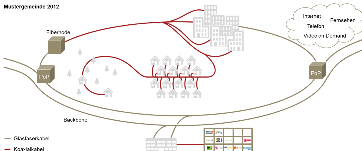
Abbildung 16: Beispielhafte Struktur eines HFC-Netztes [15].
