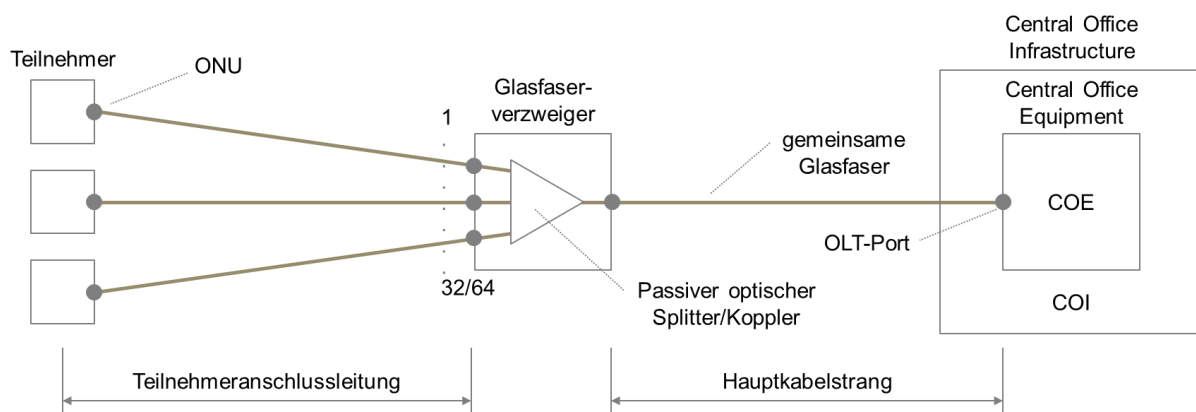
Abbildung 22: Schematische Darstellung einer GPON Strecke, [19].
