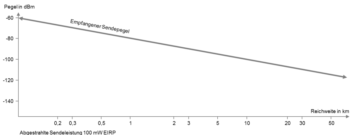
Abbildung 29: Darstellung des Signalpegels unter Berücksichtigung der Freiraumdämpfung [23].
